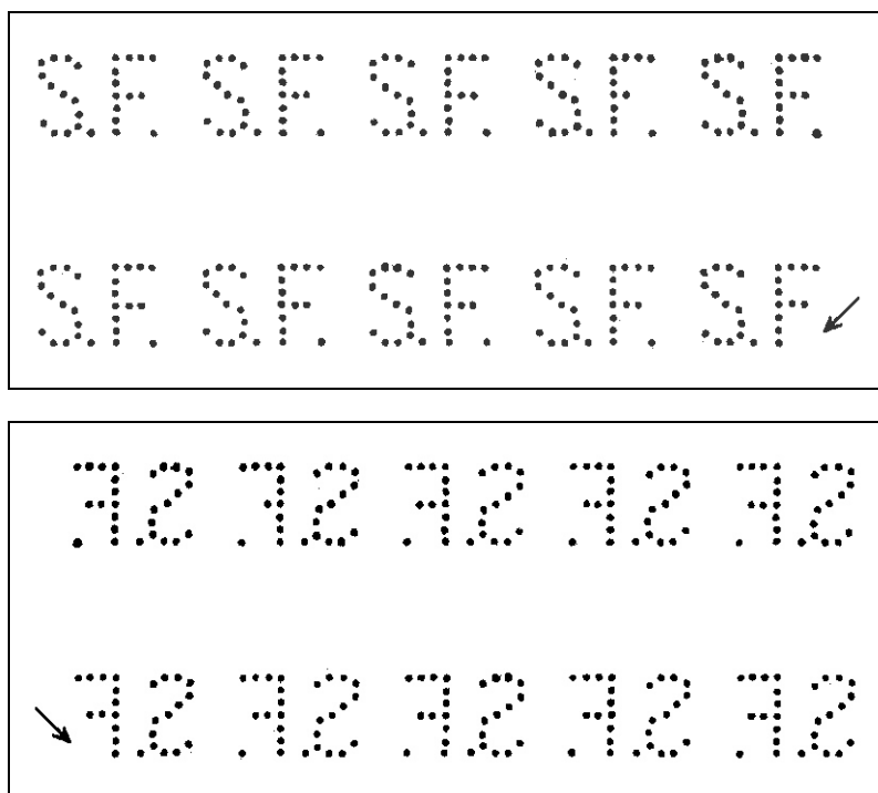
Perfinbilledet S 26. Manglende nåle markeret med pile
